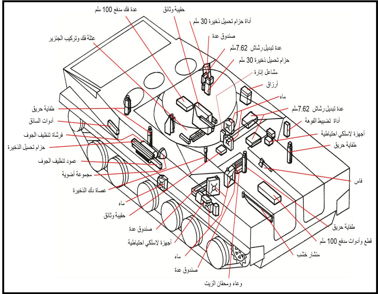
الشكل رقم (35) خطة التحميل داخل ناقلة الجنود بي ام بي - 3 (مثال)
