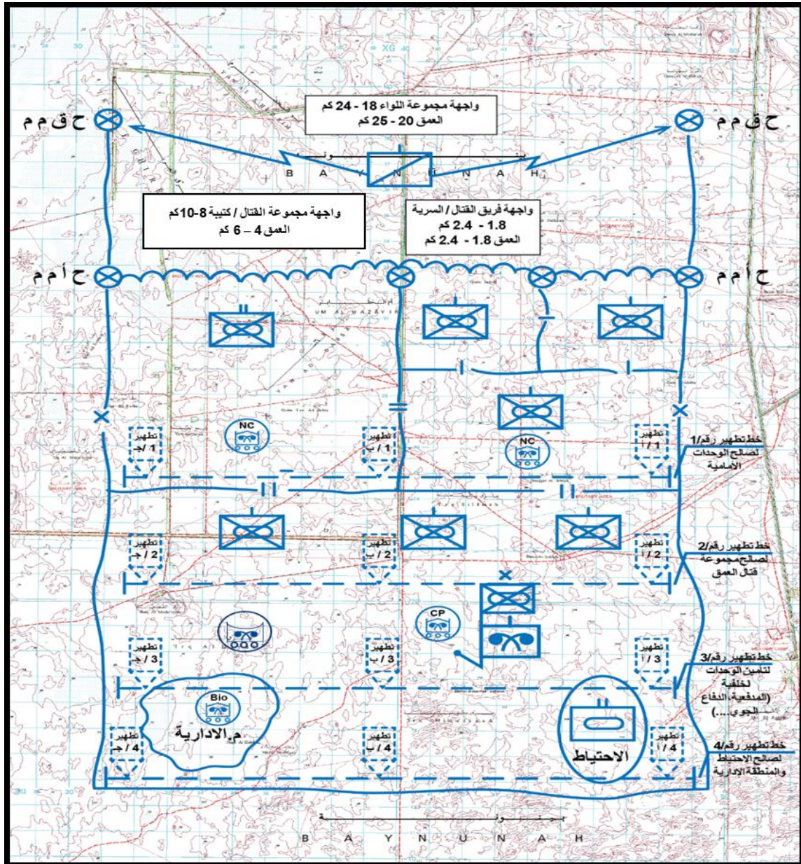
الشكل رقم (66) توزيع خطوط ومناطق التطهير في العملية الدفاعية
