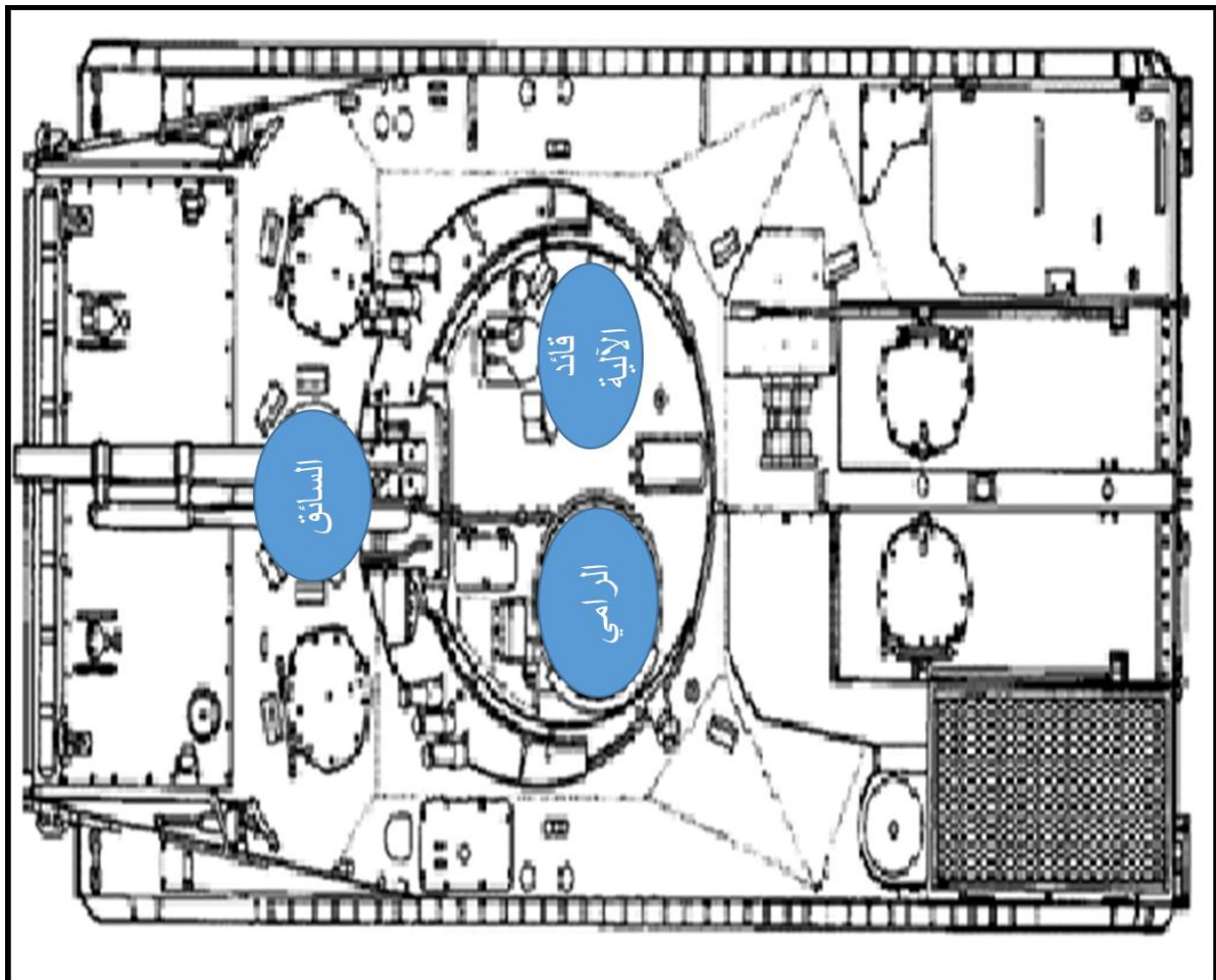
الشكل رقم (44) نموذج ناقلة بي إم بي 3 الخارجي
