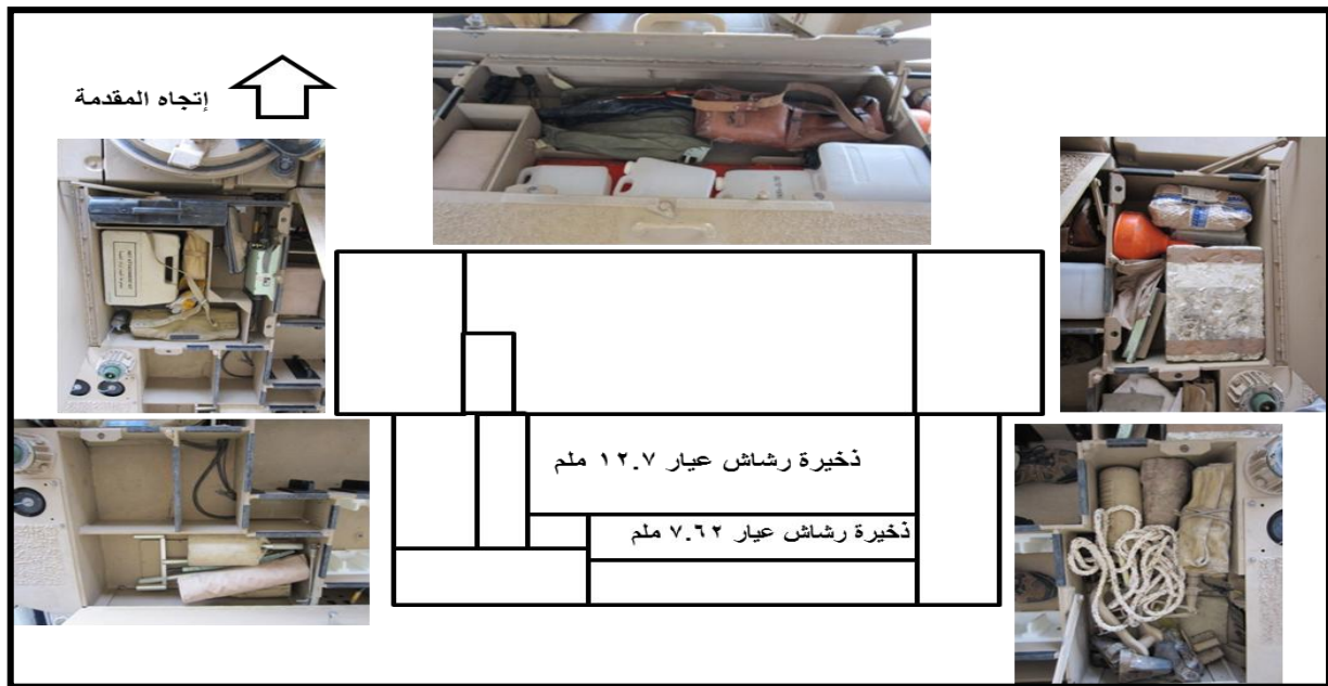
الشكل رقم (40) صناديق التخزين الخلفية لدبابة لوكيرك
