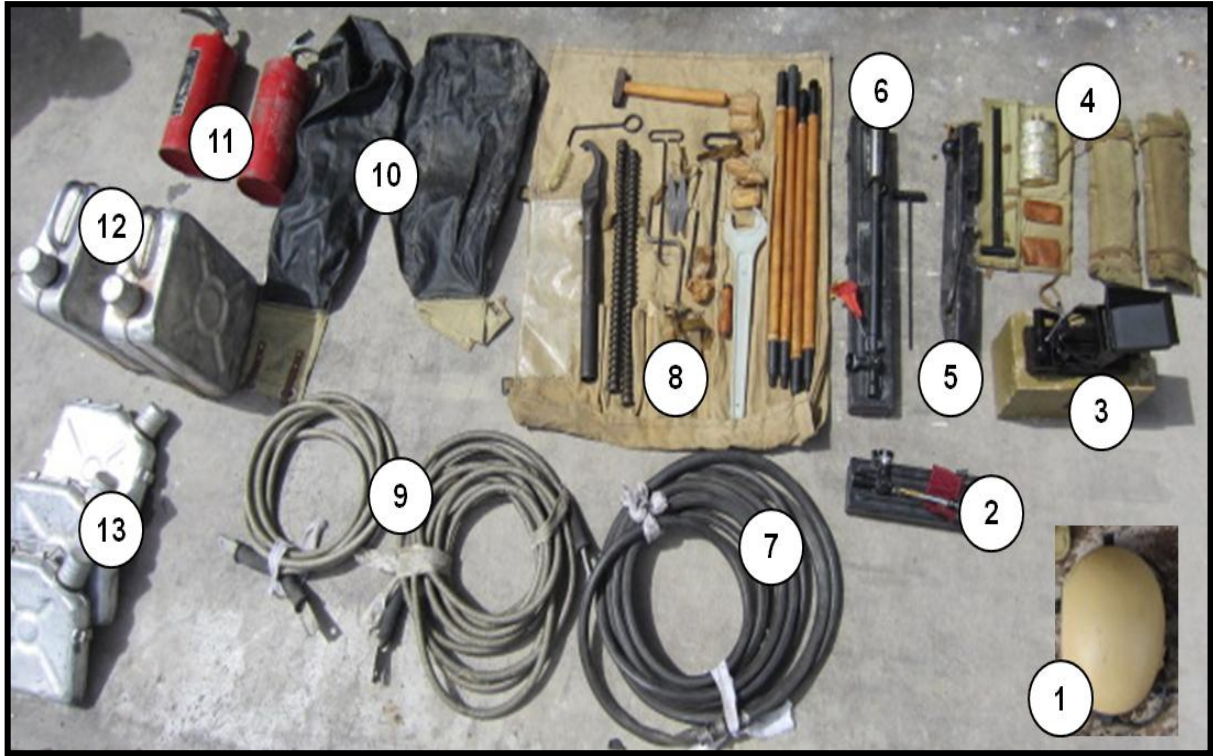
الشكل رقم (36) المجموعة الأولى من معدات ناقلة بي إم بي 3 (مثال)
