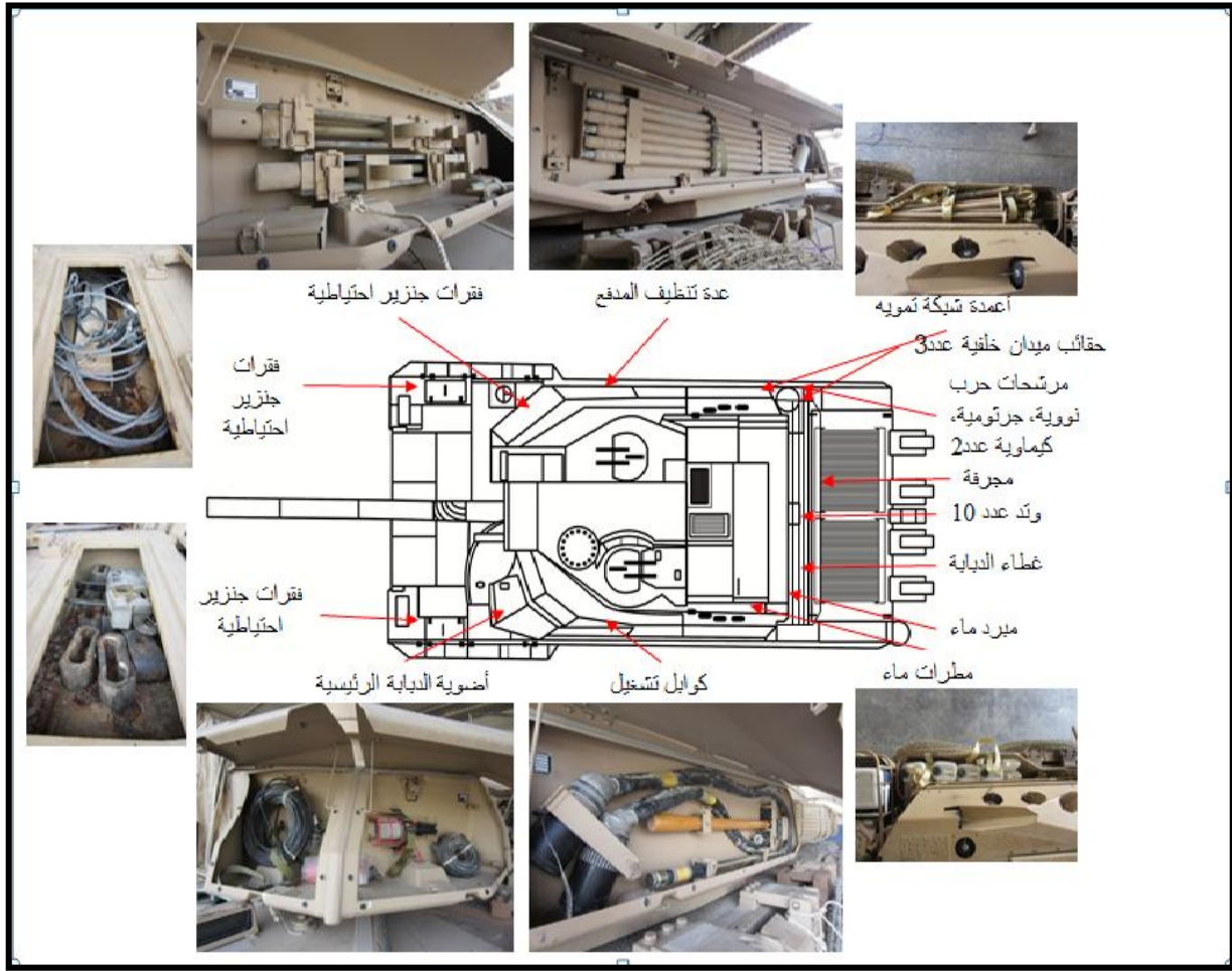
الشكل رقم (39) التخزين الخارجي لدبابة لوكيرك
