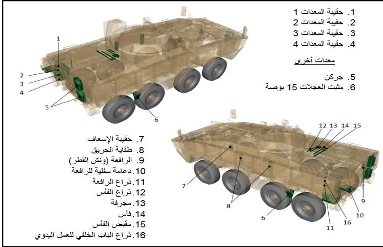
الشكل رقم (32) يرمز إلى مقرات العدة في الآلية
